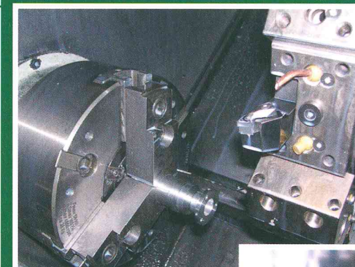
Tornio a controllo numerico "DMG MORI NLX 2500/400"
